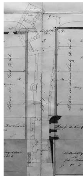
Výřez z plánů – zaměření Červené brány a přilehlého barbakánu z poloviny 19. století, Městské muzeum Horažďovice
