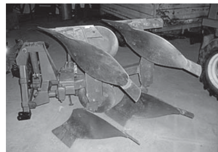
pluh APO 150 dvouradliční obracecí – nesený rok výroby 1990, nepoužívaný cena: 29 000 Kč
