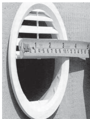
správně upravený vletový otvor v zateplené zdi
