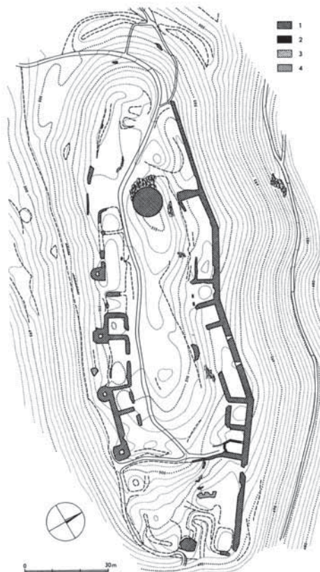
Prácheň. Půdorys hradu podle zaměření ARÚ ČSAV Praha. 1 – zdivo z počátku 14. století, 2 – zdivo poustevnické kaple vestavěné do zříceniny, 3 – destruívané bloky zdiva, 4 – na sucho skládané tarasy.
